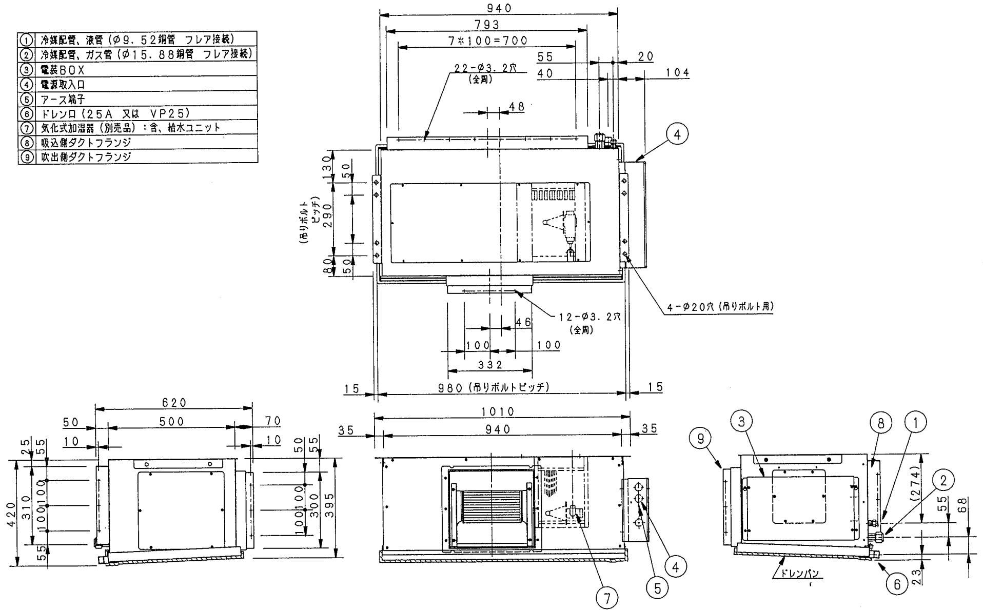
室内ユニット(天埋形) 外形寸法図 ARHZP1122SA
